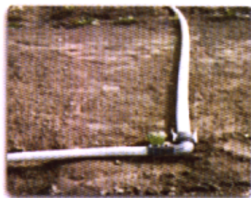
Fig. 59. a. Utilización del codo 90^\circ y b. Protección de los laterales.
