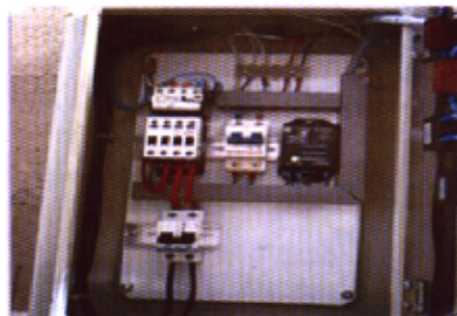
Fig. 65. Cajas con mecanismos eléctricos de protección.
